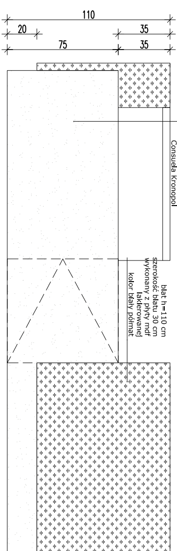
WIDOK B-B
